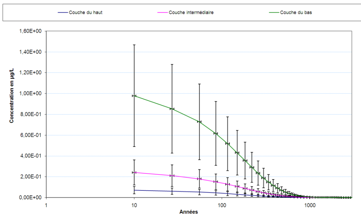
Figure 10 : Chronique des concentrations calculées pour le mercure sur le puits Amélie 1 (pour un épandage par 5 puits dans 500 ans, incertitude \pm 50\% , échelle semi-log, origine du temps prise à 500 ans)
