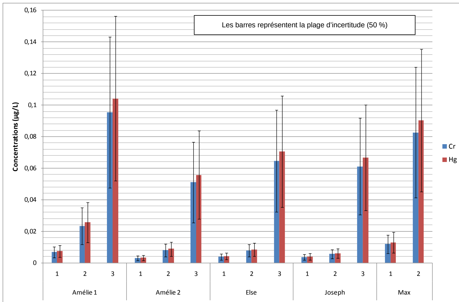
Figure 8 : Concentrations calculées en Hg (critères : 0,2 et 1 µg/L) et Cr (critères : 7 et 50 µg/L) après épandement en nappe de la saumure contaminée dans les 3 couches des 5 puits de la mine Amélie (sortie dans 1000 ans, incertitude 50 %)
