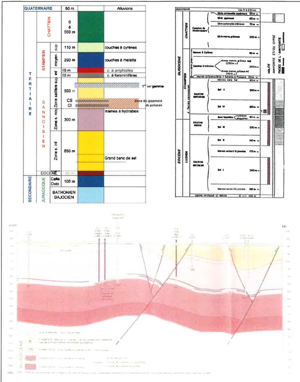
Figure 2 : Coupes géologiques des terrains aux MDP A
