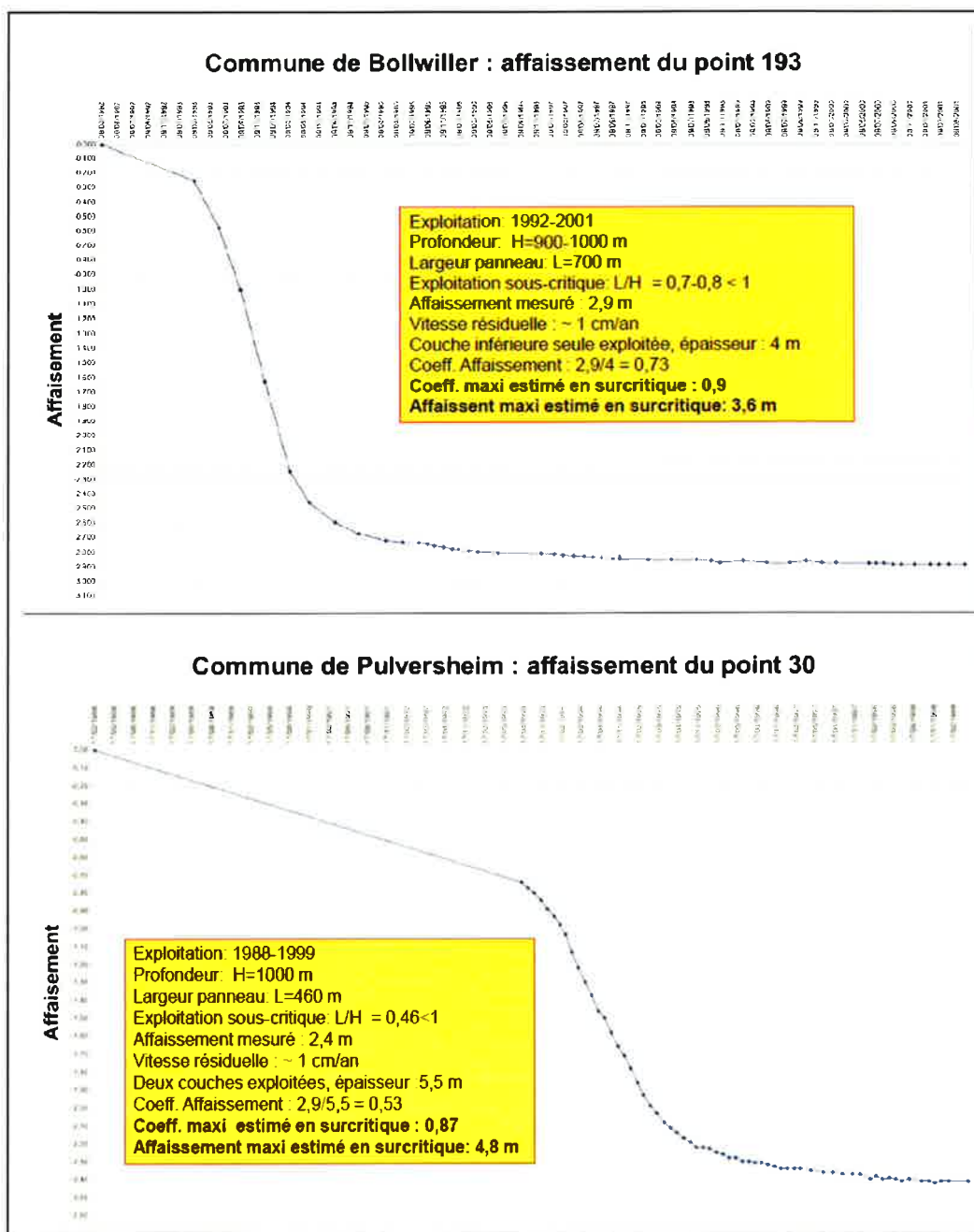
Figure 24 : Exemples d'évolution dans le temps d'affaissement lié à l'exploitation des MDPA (affaissement en m).
