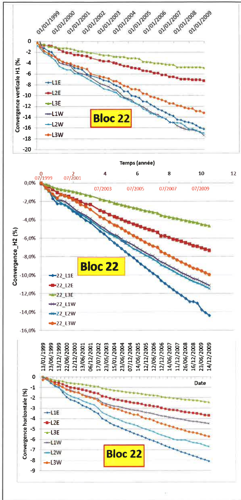
Figure 9 : Exemples des mesures de convergence dans le temps (Bloc 22, en haut : convergence verticale sur la moitié supérieure (H1), au milieu : entre le toit et le mur (H2) et en bas : convergence horizontale).
