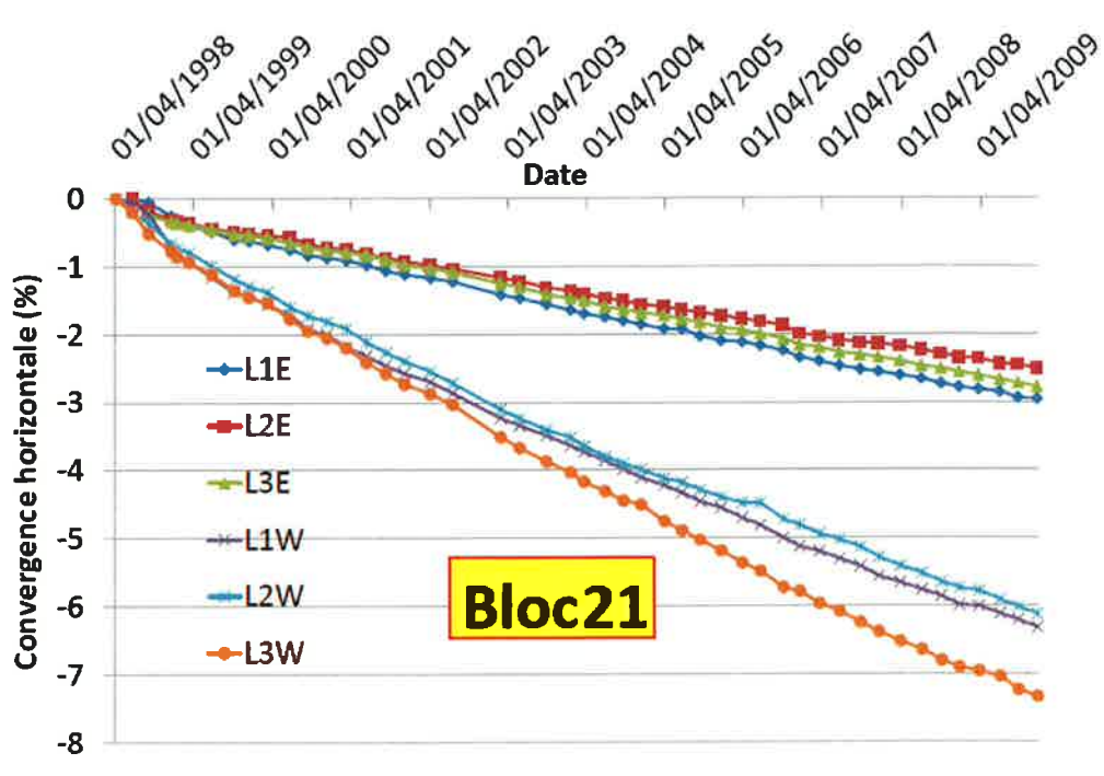
Figure A6 : Convergences horizontales (LAR) dans les blocs 11 et 21 (premiers blocs)
