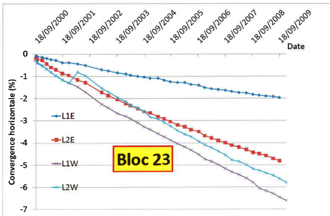
Figure A8 : Convergences horizontales (LAR) dans les blocs 13 et 23
